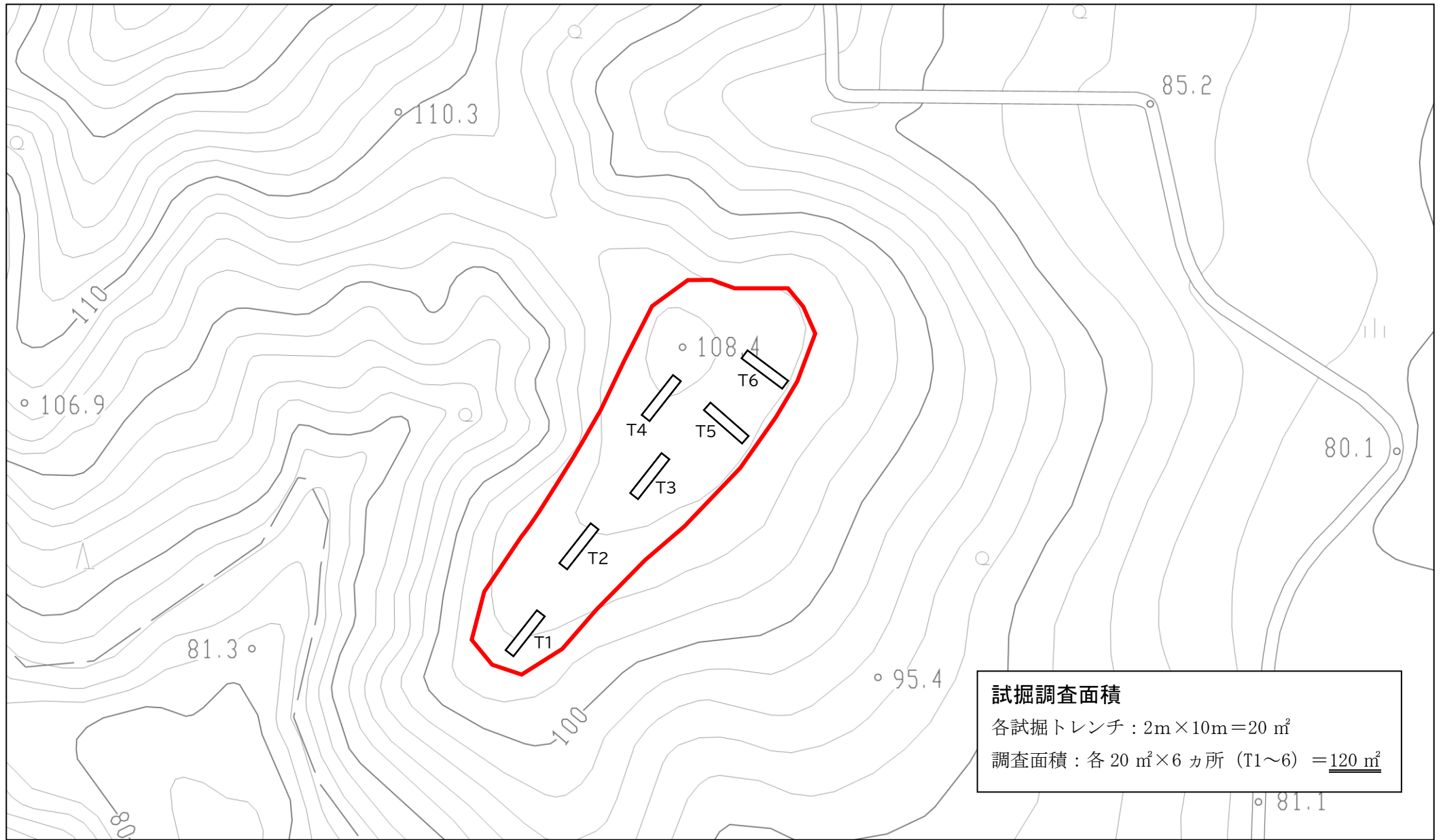
末森地区埋蔵文化財試掘確認調査 試掘トレンチ配置図
