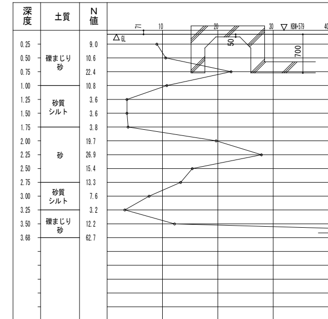
S-2 スウェーデン式サウンディング試験
