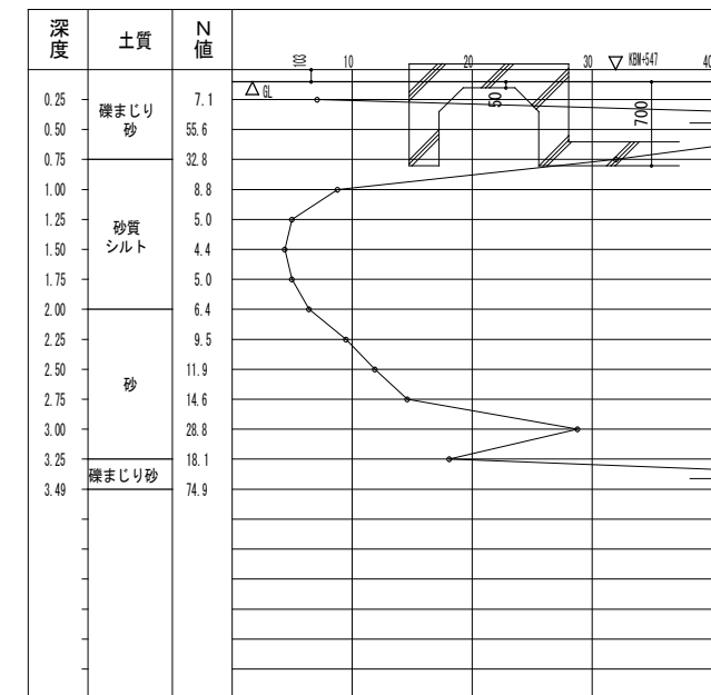
S-5 スウェーデン式サウンディング試験
