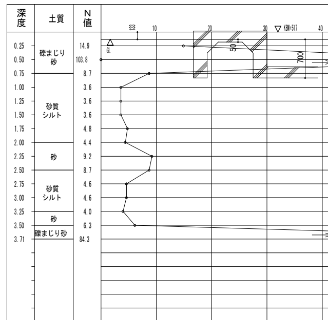
S-3 スウェーデン式サウンディング試験
