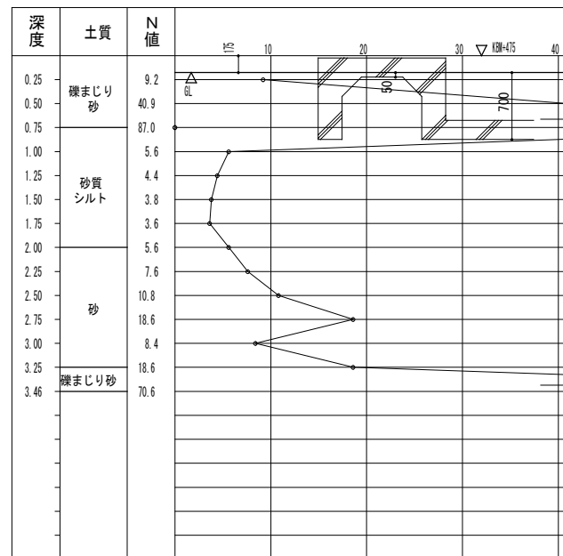
S-4 スウェーデン式サウンディング試験
