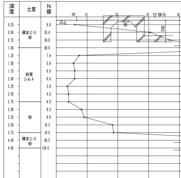
S-1 スウェーデン式サウンディング試験
