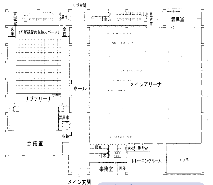
地域スポーツセンター平面図
