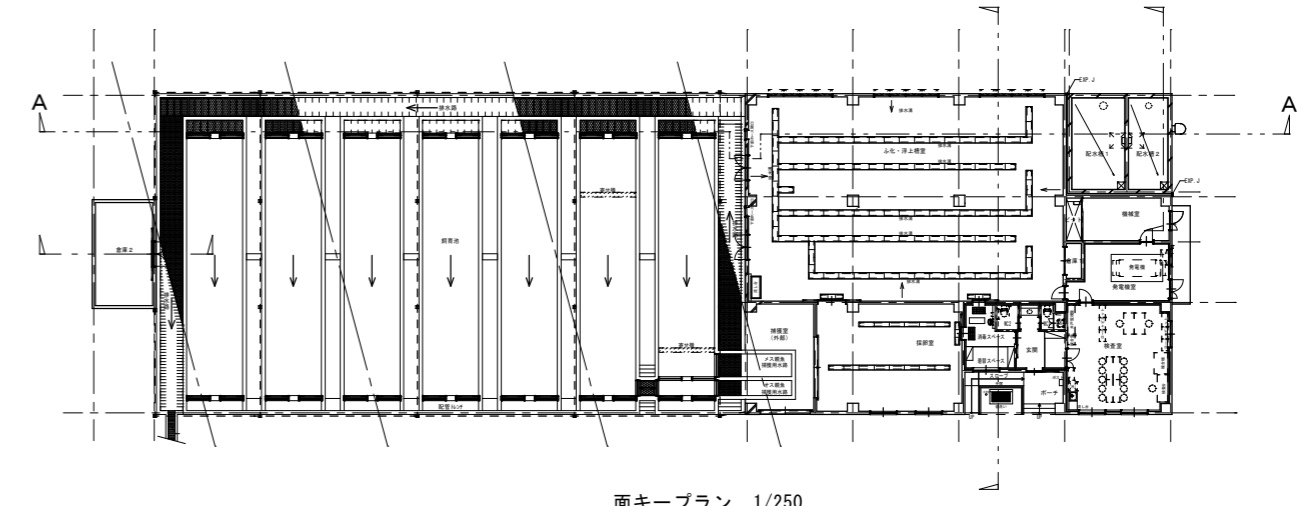
面キープラン 1/250
