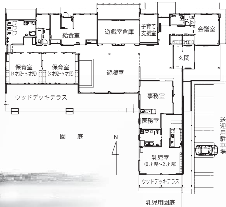
浪江認定こども園(仮称)平面図
