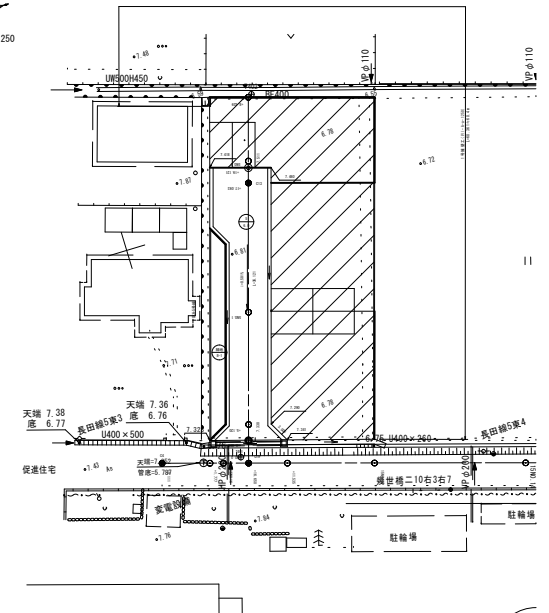
造成計画平面図 (2/2) (1工区・隔地)
