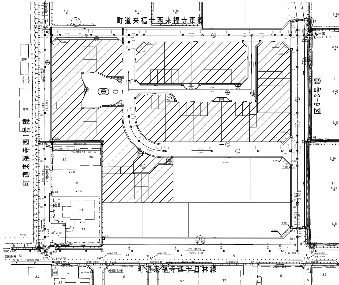
造成計画平面図 (1/2) (1工区・南)
